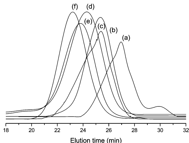
Figure 7. GPC traces of neutralized polymers: (a) poly(AP- g -PEO-750), (b) polyaniline, (c) poly((AP- g -PEO-750)- co -aniline) (6/1), (d) poly((AP- g -PEO-750)- co -aniline) (1/1), (e) poly((AP- g -PEO-350)- co -aniline) (3/1), and (f) poly((AP- g -PEO-750)- co -aniline) (3/1).
